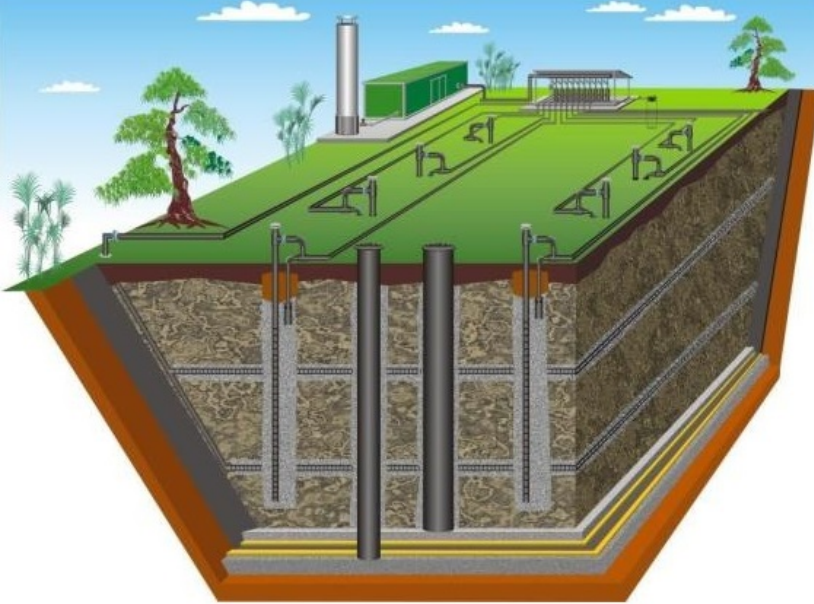
Resim 1: Katı atık depolama sahası (şematik)
